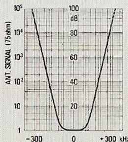
Selectiviteits karakteristiek van de FM-ontvanger.
